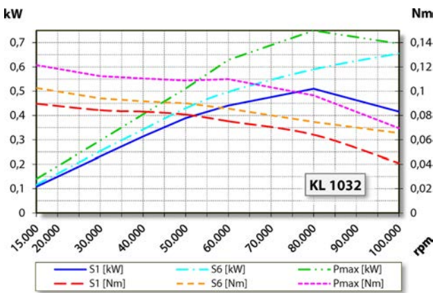
Leistungsdiagramm Spindelträgerkühlung
