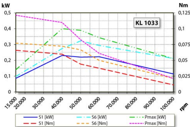
Leistungsdiagramm Druckluftgekühlt
