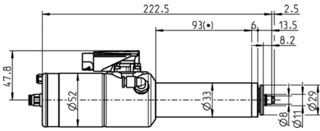
寸法図
