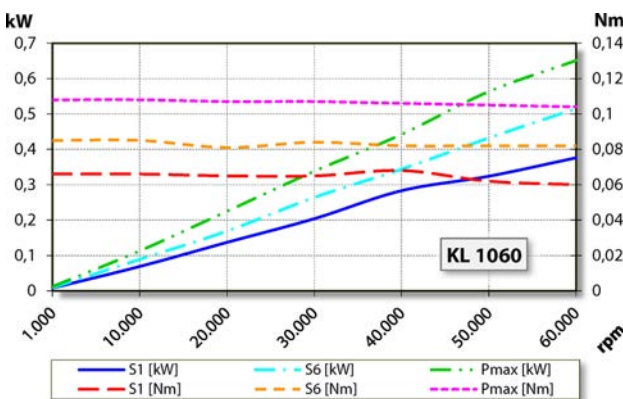
出力、トルク-回転数ダイアグラム 無冷却
