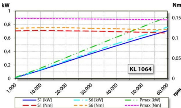
出力、トルク-回転数ダイアグラム スピンドルホルダー冷却
