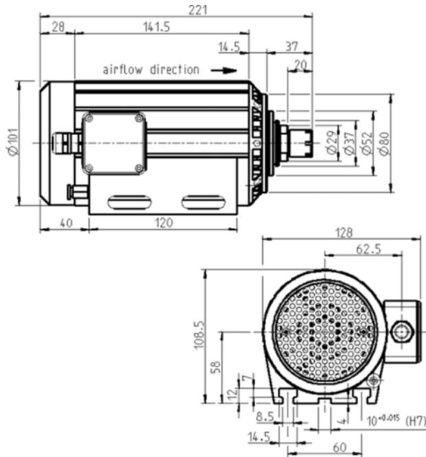
寸法図
