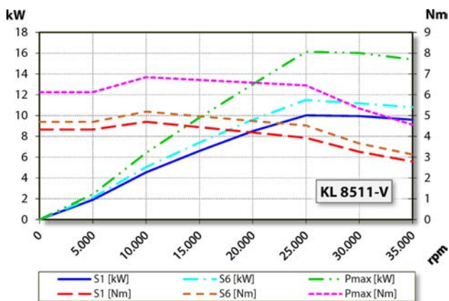
Leistungsdigramm Flüssigkeitsgekühlt
