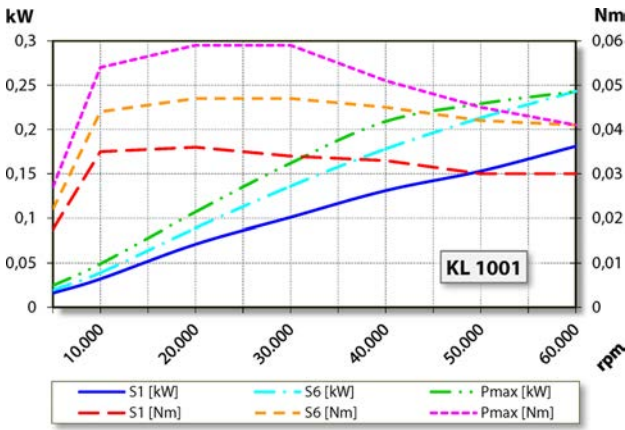
Güç diyagramı Soğutulmamış
