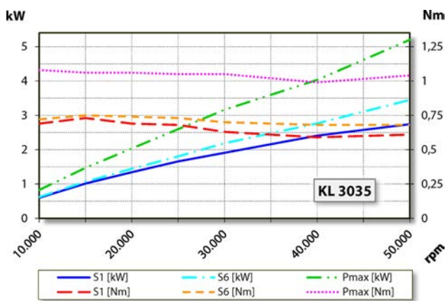
Leistungsdigramm
